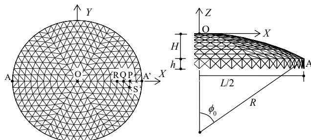
図1 解析モデル
